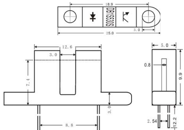
图.6 外形尺寸图 (单位: 毫米 ±0.1)
